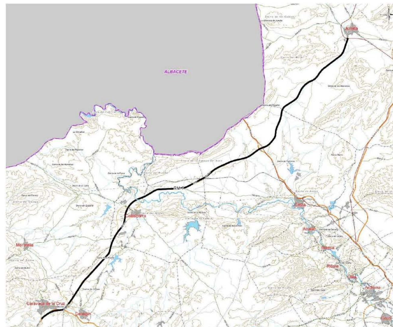
Infraestructuras propuestas. Autovía Jumilla - Caravaca (RM-7)
