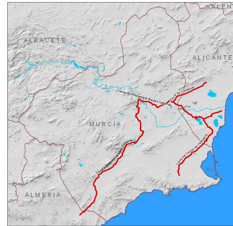
Figura 1.25. Planta general de los Canales Post-Trasvase (Fuente: Elaboración propia)
