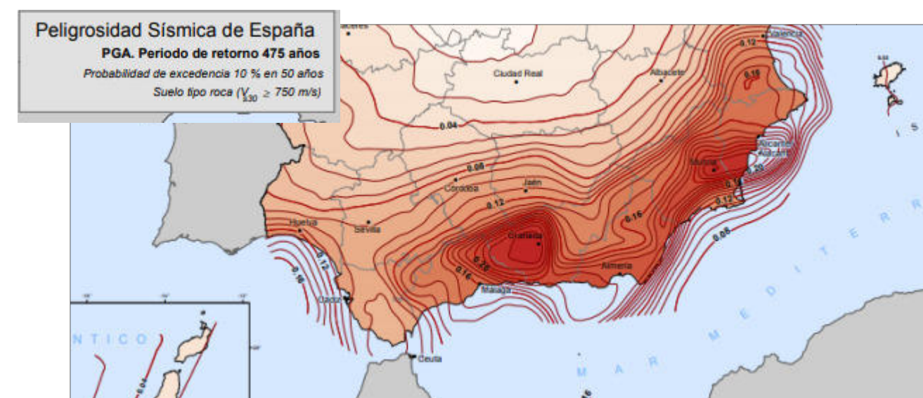
Mapa de peligrosidad sísmica. Fuente: IGN. Año 2015
