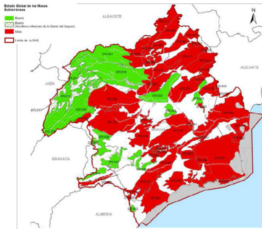
Estado global de las masas subterráneas. Fuente CHS
