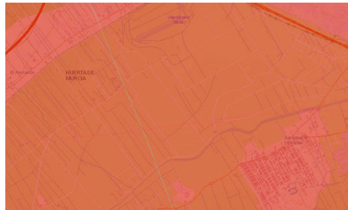
Valor histórico del Ozono Troposférico. Fuente: Ministerio para la transición ecológica
