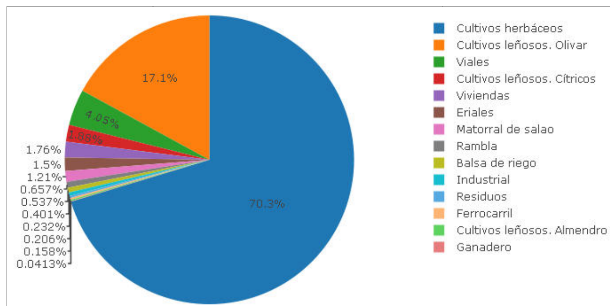
Suelos en relación a la ZAL. Fuente: Mapa de Suelos Región de Murcia
