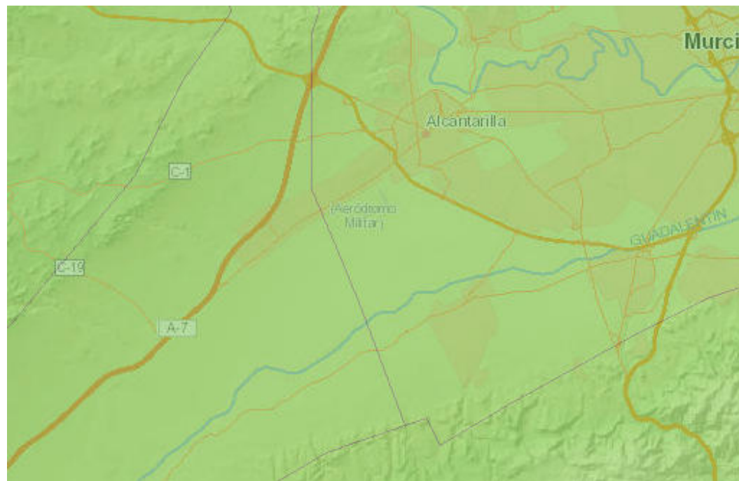
Valor histórico de PM 2,5 . Fuente: Ministerio para la transición ecológica y elaboración propia
