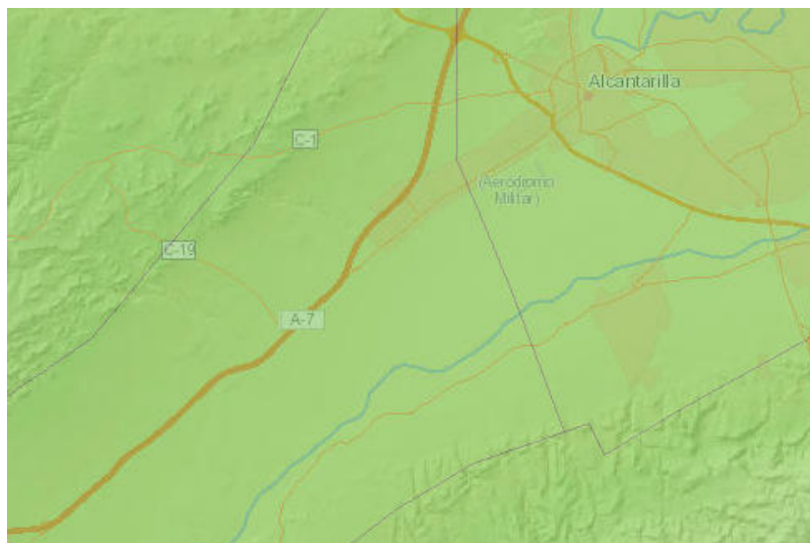
Valor histórico de SO 2 . Fuente: Ministerio para la transición ecológica y elaboración propia
