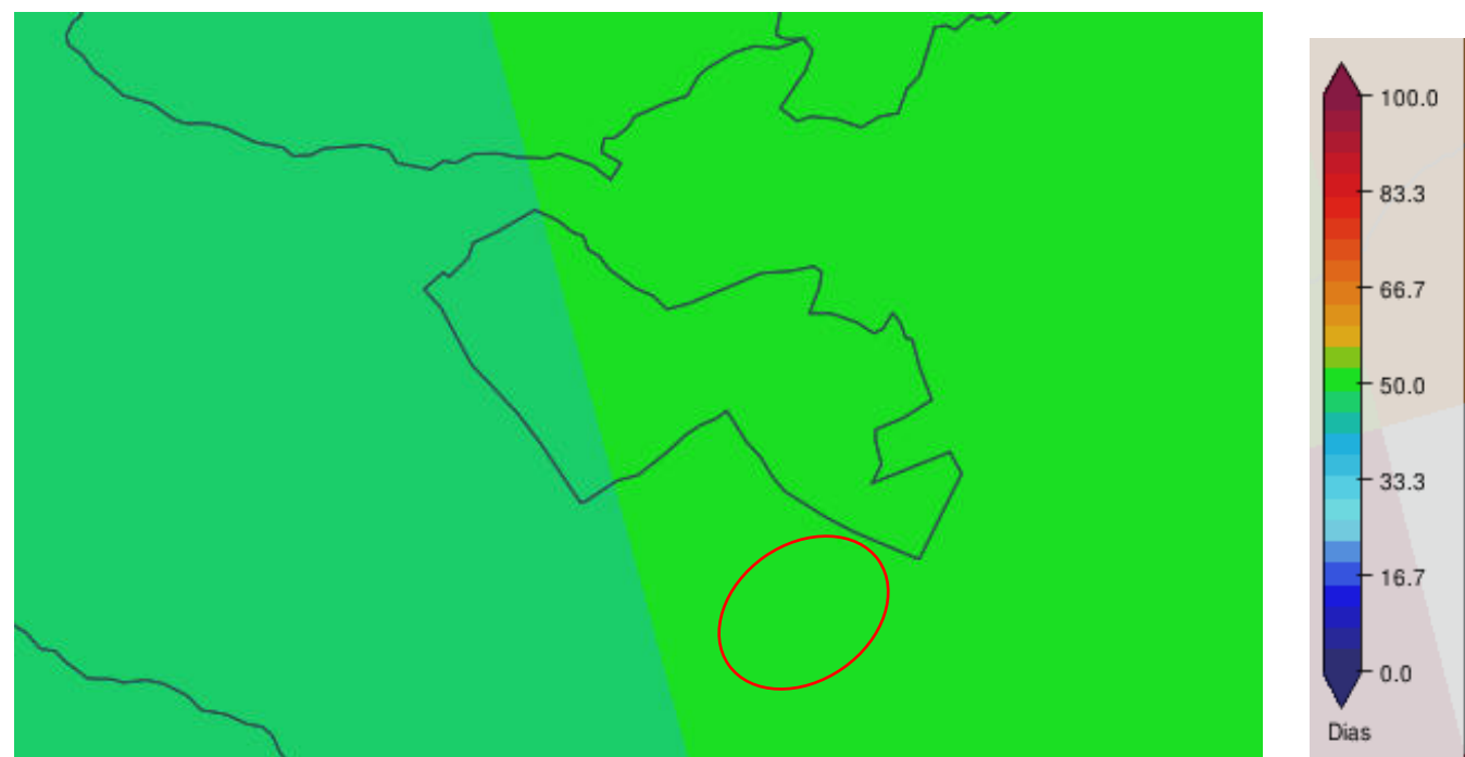
Nº de días con temperatura mínima > 20°C. Futuro cercano 2011-2040
