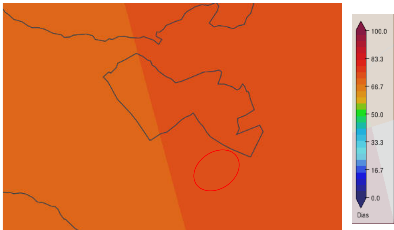
Nº de días con temperatura mínima > 20°C. Futuro medio 2041-2070
