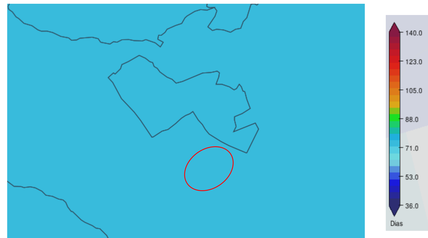
Número de días cálidos. Futuro medio 2041-2070
