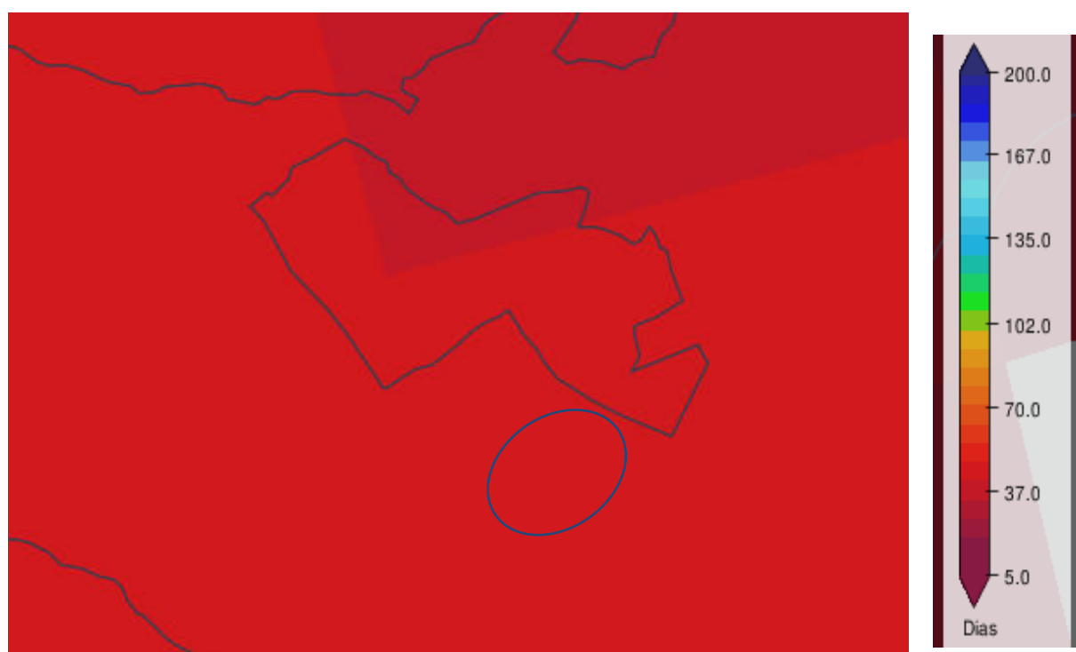
Número de días de lluvia. Futuro cercano 2011-2040
