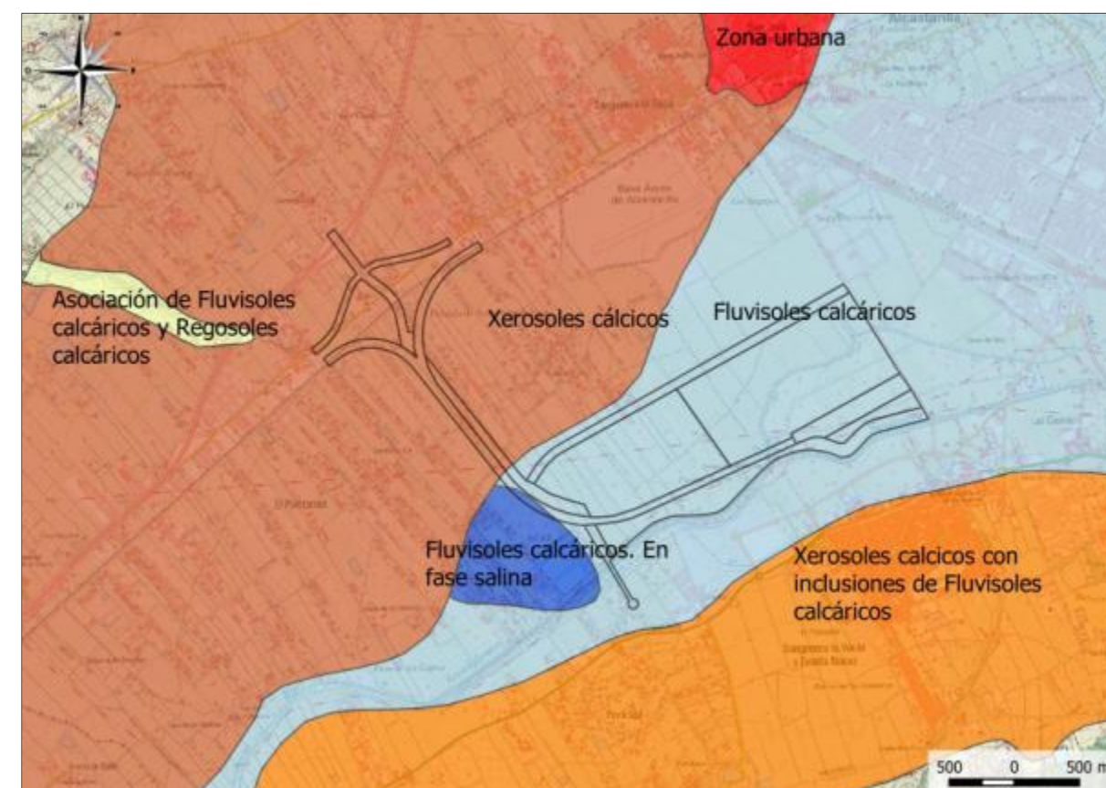
Suelos en relación a la ZAL. Fuente: Mapa de Suelos Región de Murcia
